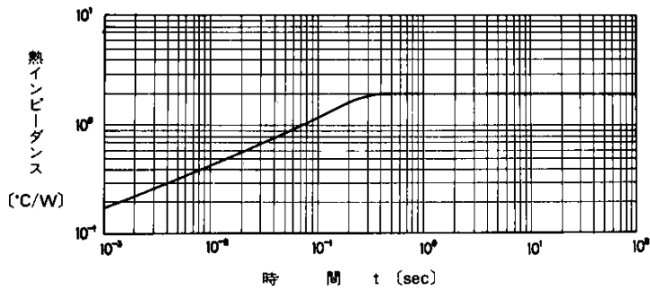
時間 t (sec) 過渡熱インピーダンス Transient Thermal Impedance
