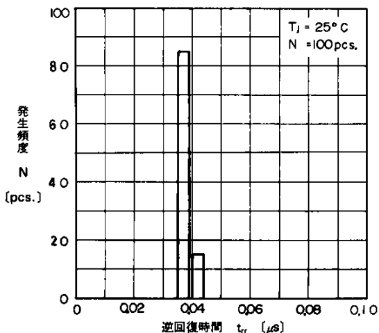
逆回復時間特性分布 (代表特性) Reverse Recovery Time
