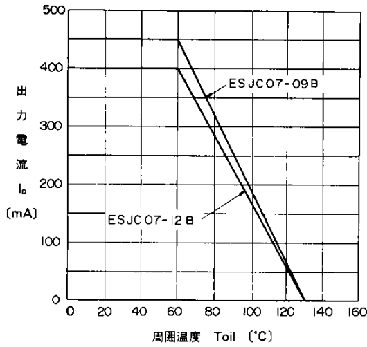
電流低減特性曲線 Current Derating Curve
