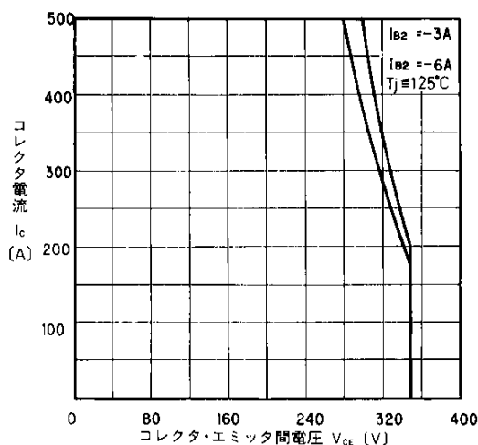
安全動作領域(逆バイアス)
