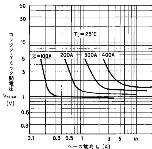
出力特性
