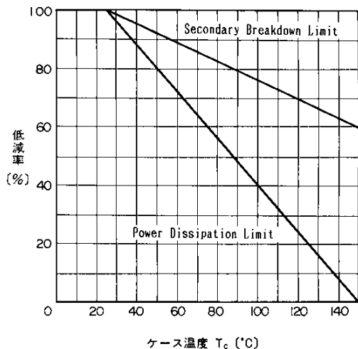
ケース温度 T_c ( ^\circ C ) ASO 低減特性 ASO Derating
