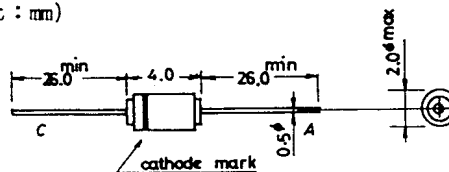
外形図 1080 (unit: mm)
