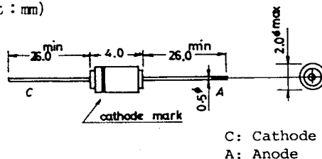
外形図 1080 (unit: mm)
