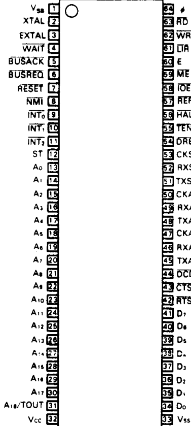
(DP-64S)
