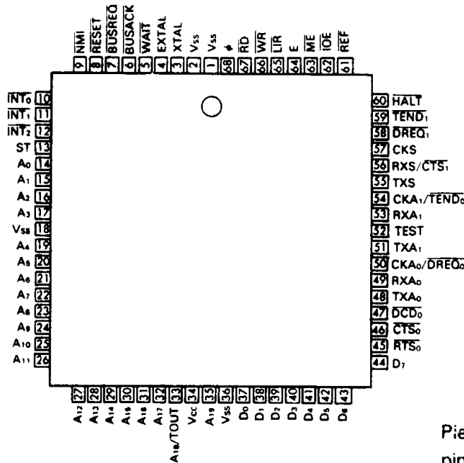
(CP-68)
