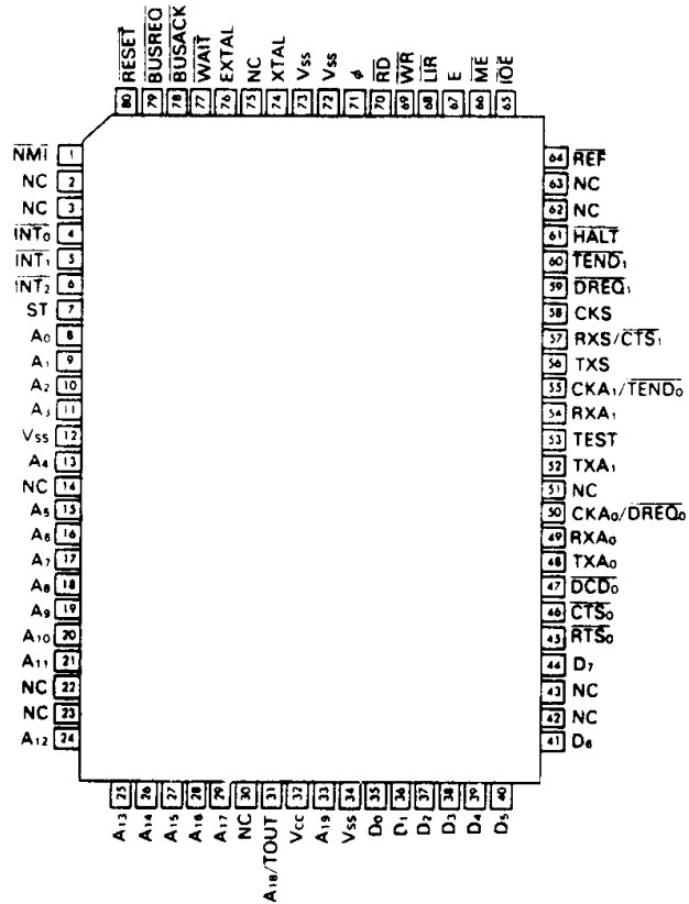
(FP-80B)
