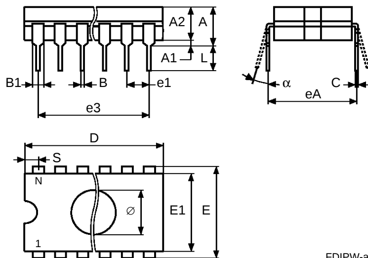
FDIPW-a
