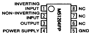
Outline 8P2S-A
