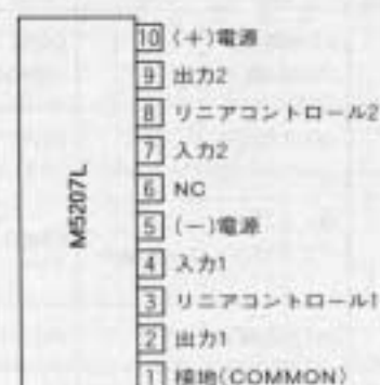
外形 10P5
