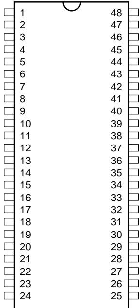
48 Pin SSOP
