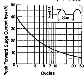
IFSM Characteristics (EK03.04)
