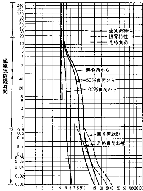
平均順電流 I_{F(AV)} (A) 過負荷電流—時間 (冷却体AE01-6) 自冷 周囲温度 40° 50Hz正弦半波電流 (通流角180°)
