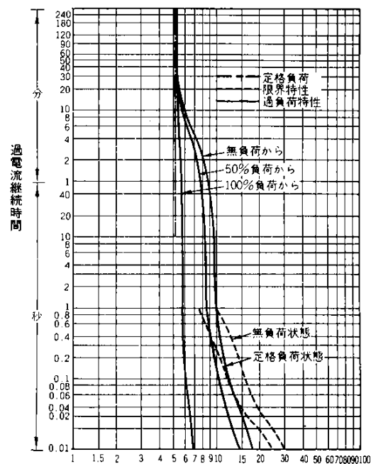
電流波高値( \times 10 ) (A) 過負荷電流—時間 (冷却体AG01-6B) 自冷 周囲温度 40° 50Hz正弦半波電流 (通流角180°)
