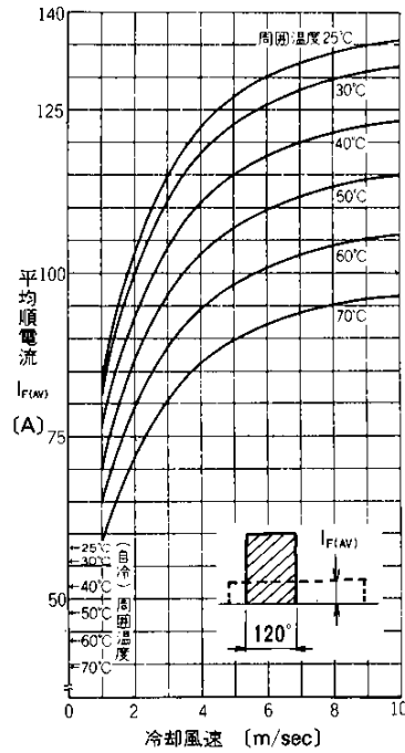
平均順電流—冷却風速 (方形波120°導通, 冷却体AH02-12)
