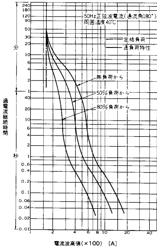
過負荷電流—時間 (冷却体AH01-12B自冷)
