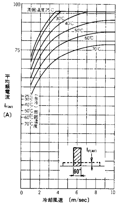
平均順電流—冷却風速 (方形波60°導通, 冷却体AH02-12)
