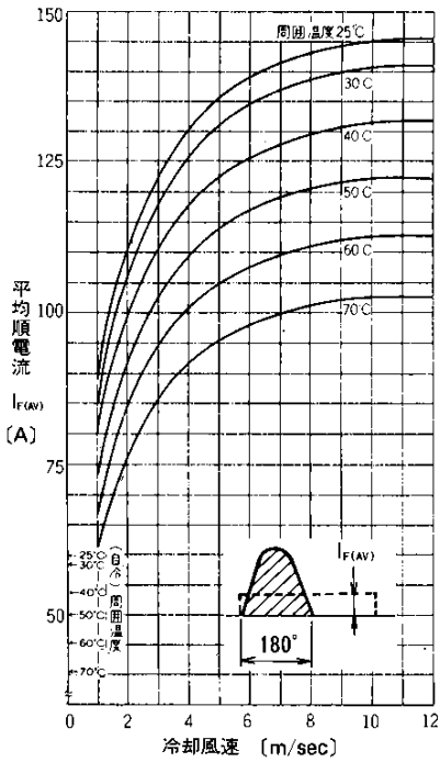
平均順電流—冷却風速 (正弦波180°導通, 冷却体AH02-12)
