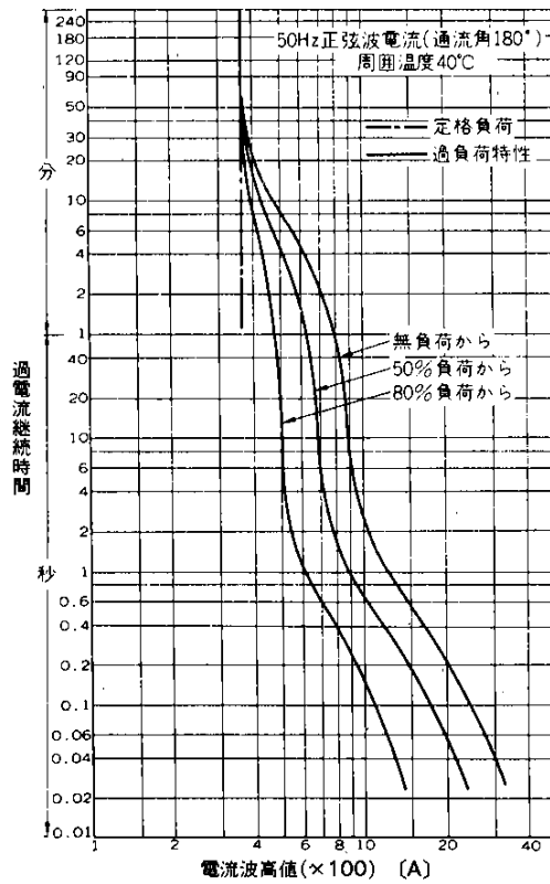
過負荷電流—時間 (冷却体AL01-20自冷)
