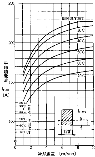
平均順電流—冷却風速 (方形波120°導通, 冷却体AL01-20)
