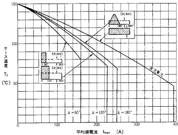
平均順電流—ケース温度
