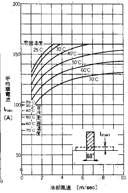
平均順電流—冷却風速 (方形波60°導通, 冷却体AL01-20)
