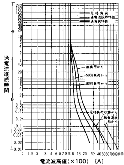
電流波高値(×100) (A) 過負荷電流—時間 (冷却体AL01-24) 風冷6m/s 周囲温度40°C50Hz正弦波電流(通流角180°)
