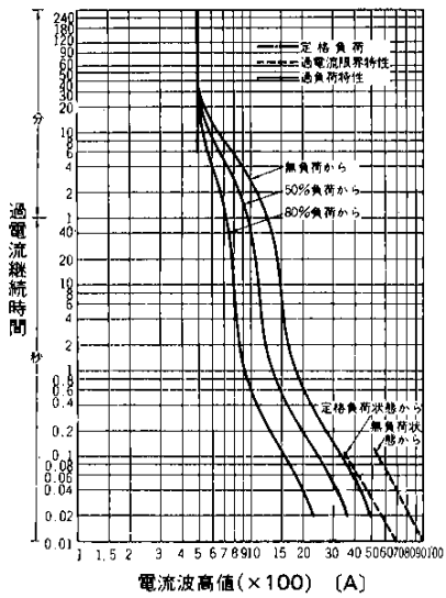
電流波高値(×100) (A) 過負荷電流—時間 (冷却体AL01-24) 自冷 周囲温度40°C50Hz正弦波電流(通流角180°)
