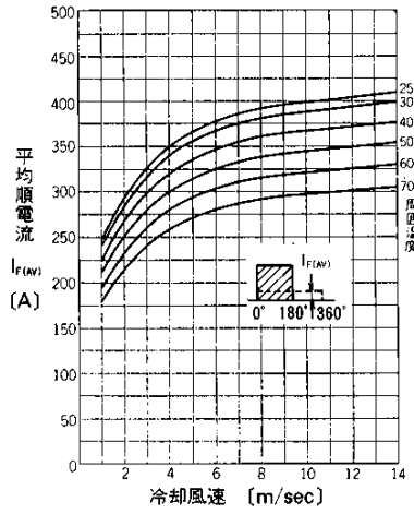
平均順電流—冷却風速 (方形波180°導通, 冷却体AL01-24)
