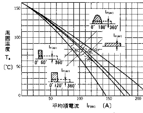
平均順電流—周囲温度 (冷却体AL01-24付) 自冷
