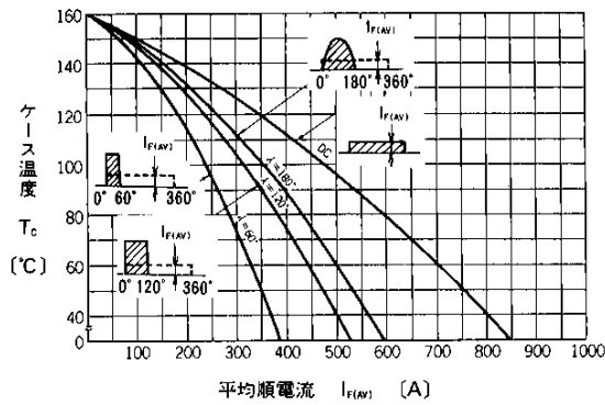
平均順電流—ケース温度
