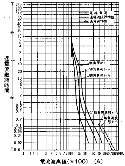
過負荷電流—時間 (冷却体AL01-24)風冷6m/s 周囲温度40°C50Hz正弦波電流(通流角180°)
