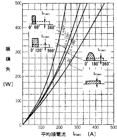
順損失
