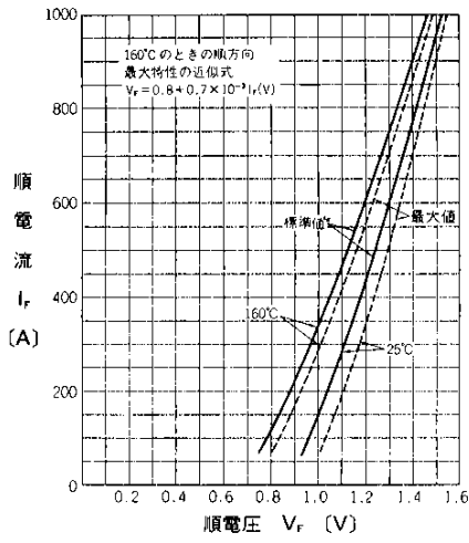
順特性
