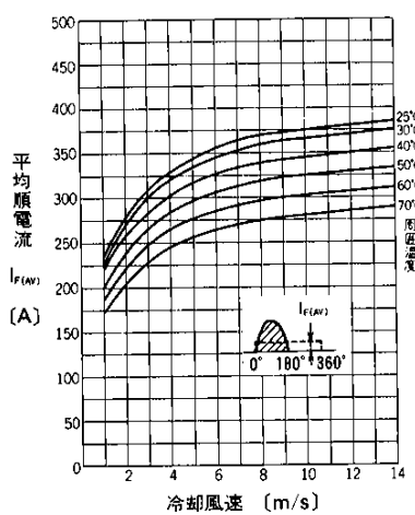
平均順電流—冷却風速 (正弦波180°導通 冷却体AL01-24)
