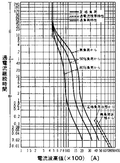
過負荷電流—時間 (冷却体AL01-24)自冷 周囲温度40°C50Hz正弦波電流(通流角180°)
