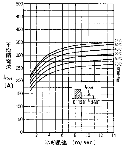
平均順電流—冷却風速 (方形波120°導通, 冷却体AL01-24)
