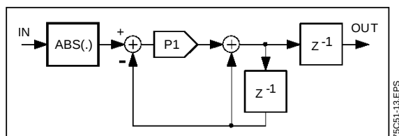
Figure G2 : Power Estimator
