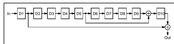
Figure 19 : Actual x^9 + x^4 + 1 Descrambler
