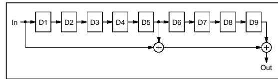
Figure 19 : Actual x^9 + x^4 + 1 Descrambler
