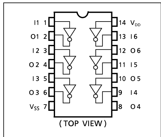
FN (SOL14-P-150-1.27) Weight : 0.12g (Typ.)
