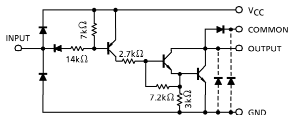
TD62387AP, TD62387AF
