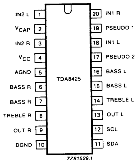
Fig. 2 Pinning diagram.
