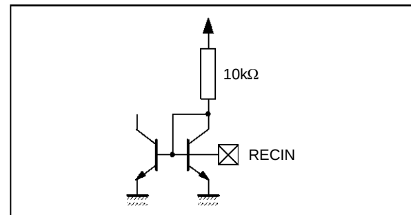
Pin : RECIN
