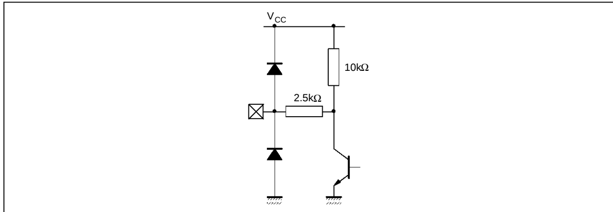
Pin : V1-SP, V2-SP, V1-LP, V2-LP
