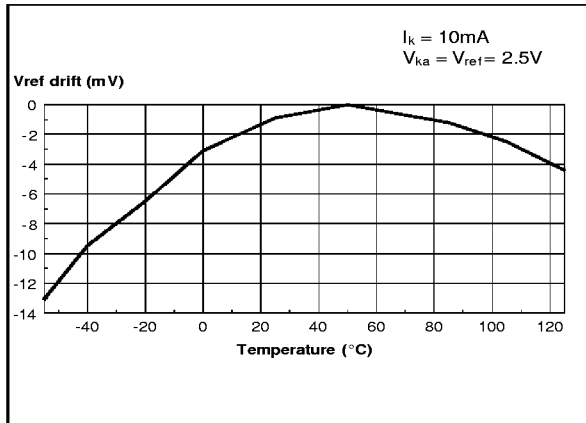
DRIFT (mV) vs TEMPERATURE (°C)
