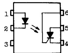
ピン接続図
