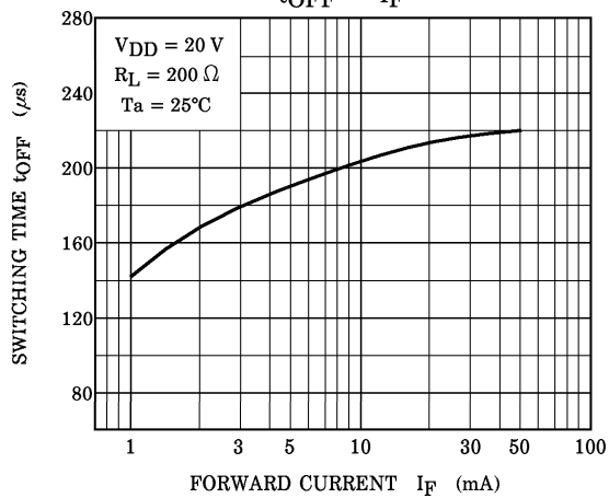
t_{OFF} - I_F
