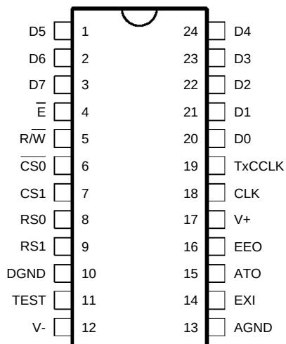
DIP24 : TS68950
