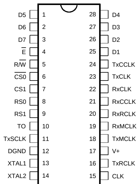
DIP28 : TS68952
