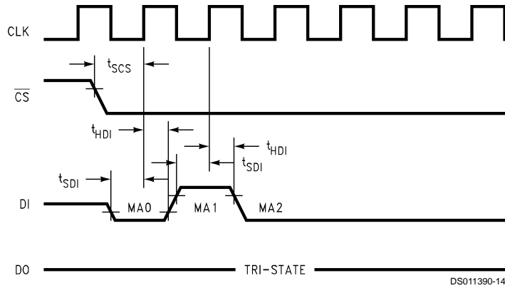
FIGURE 3. DI Timing
