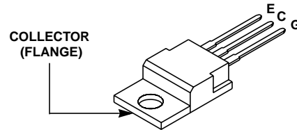
JEDEC TO-220AB
