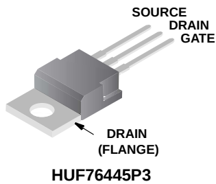
JEDEC TO-220AB
