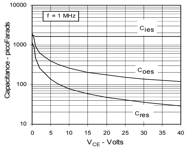
Fig. 16. Capacitance
