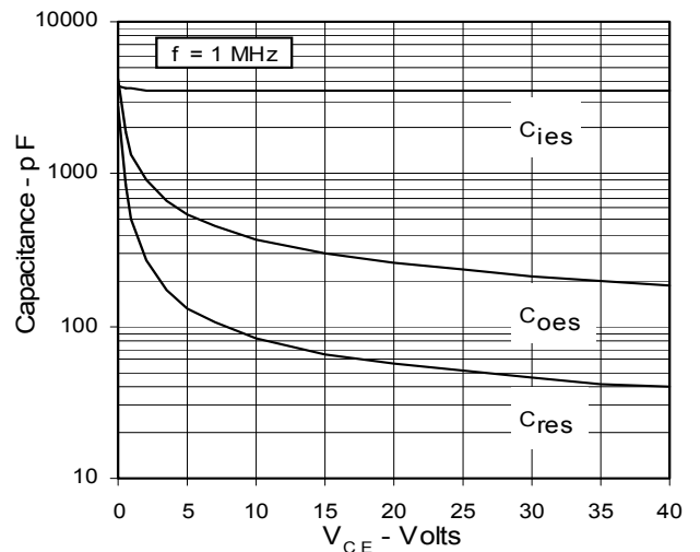
Fig. 16. Capacitance
