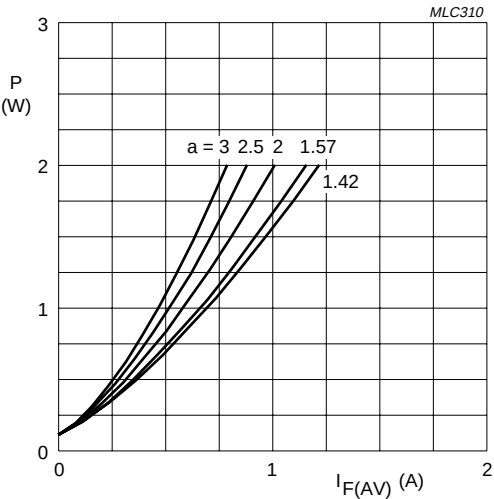
BYD43U and V a = I_{F(RMS)}/I_{F(AV)} ; V_R = V_{RRMmax} ; \delta = 0.5 .
