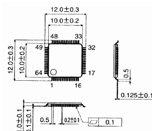
TQFP64V
