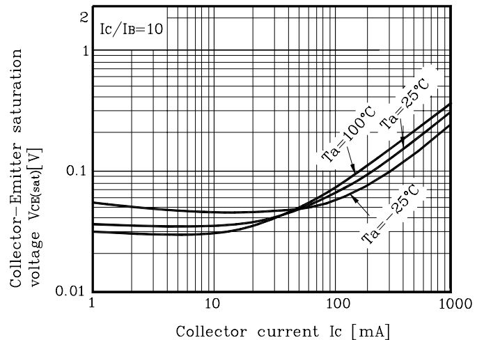
Fig. 4 V_{CE(sat)} - I_C
