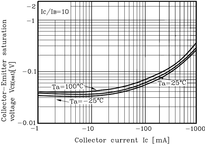
Fig. 5 VCE(sat) - IC
