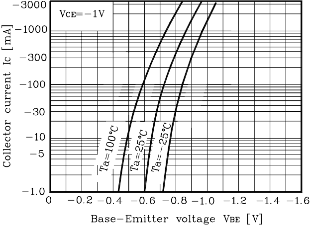
Fig. 2 IC - VBE
