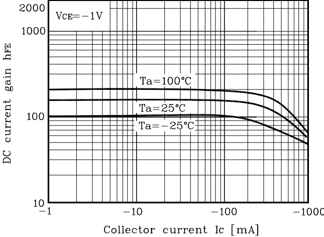
Fig. 4 hFE - IC
