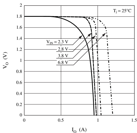
V_O - I_O
