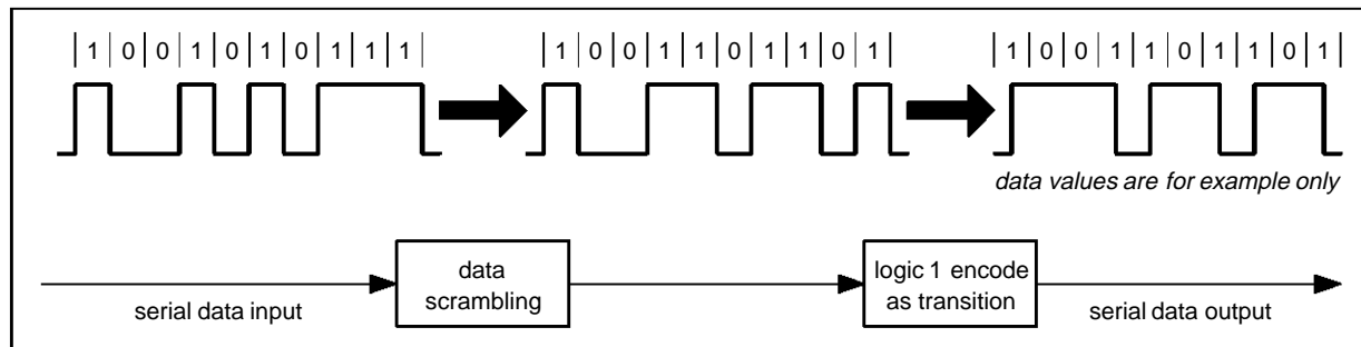
Figure 6 : Data Serialisation
