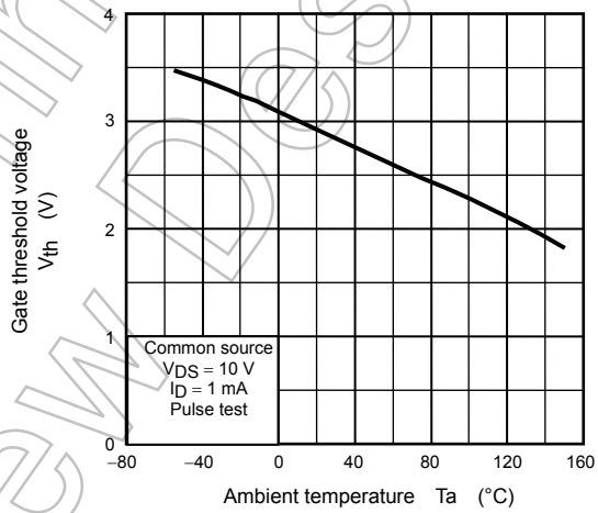
V_{th} - T_a
