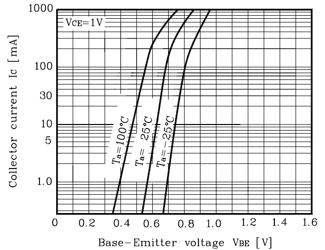
Fig. 2 I_C - V_{BE}
