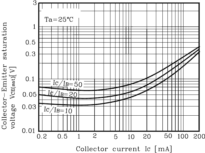
Fig. 5 V_{CE(sat)} - I_C
