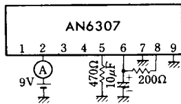
Test Circuit 1 (I tot )
