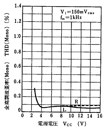
THD(Mono) - V_{CC}
