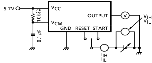
4. V_{IH} , V_{IL} , I_{IH} , I_{IL}
