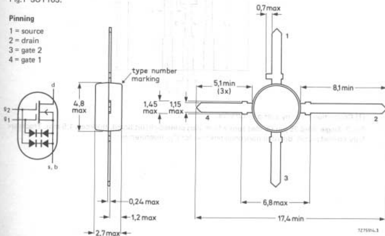
Fig.1 SOT103.
