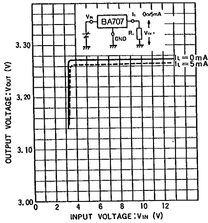
Fig.3 入出力特性
