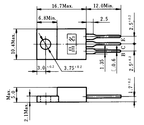
外形寸法 (単位: mm)
