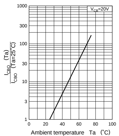
I_{CBO} - T_a
