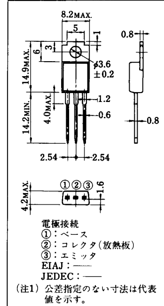
外形図
